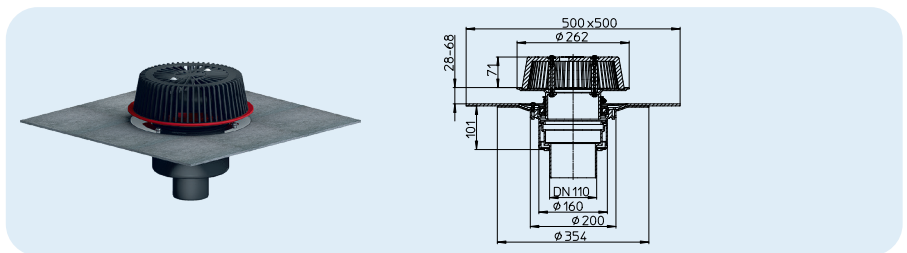
Ablaufleistung gemessen nach DIN EN 1253 mit Stutzen an Fallleitung 3 m Ablaufleistung in l/s bei Anstauhöhe 5 - 65 mm
